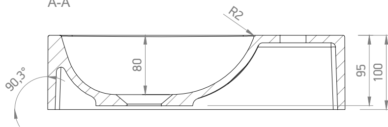
A-A
