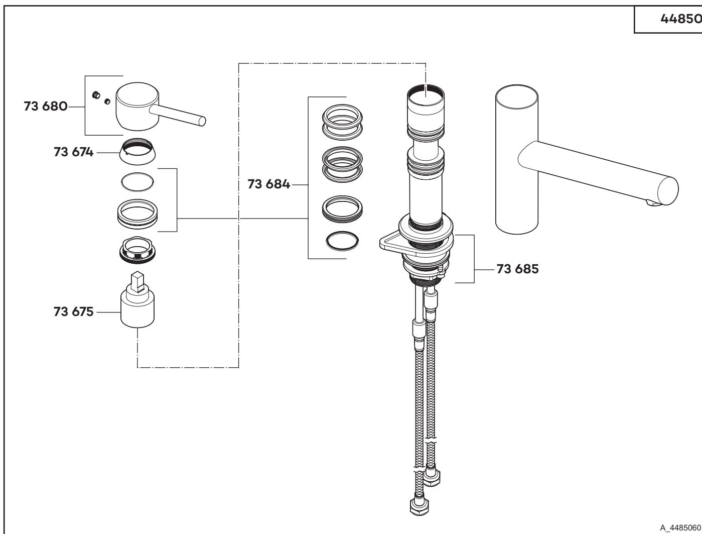
44850 Spültisch-Einhandmischer DN 15 single lever sink mixer DN 15 ééngreeps gootsteenmengkraan 1/2"
